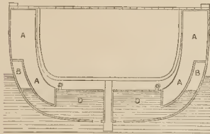
Fig. 3. Sección transversal del barco insubmersible DD Water-ballast. - A, A, A, A, B, B, cajones de aire comprimido.
